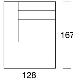
Penisola GRANDE DX/SX L. 128 P.167 H.88
